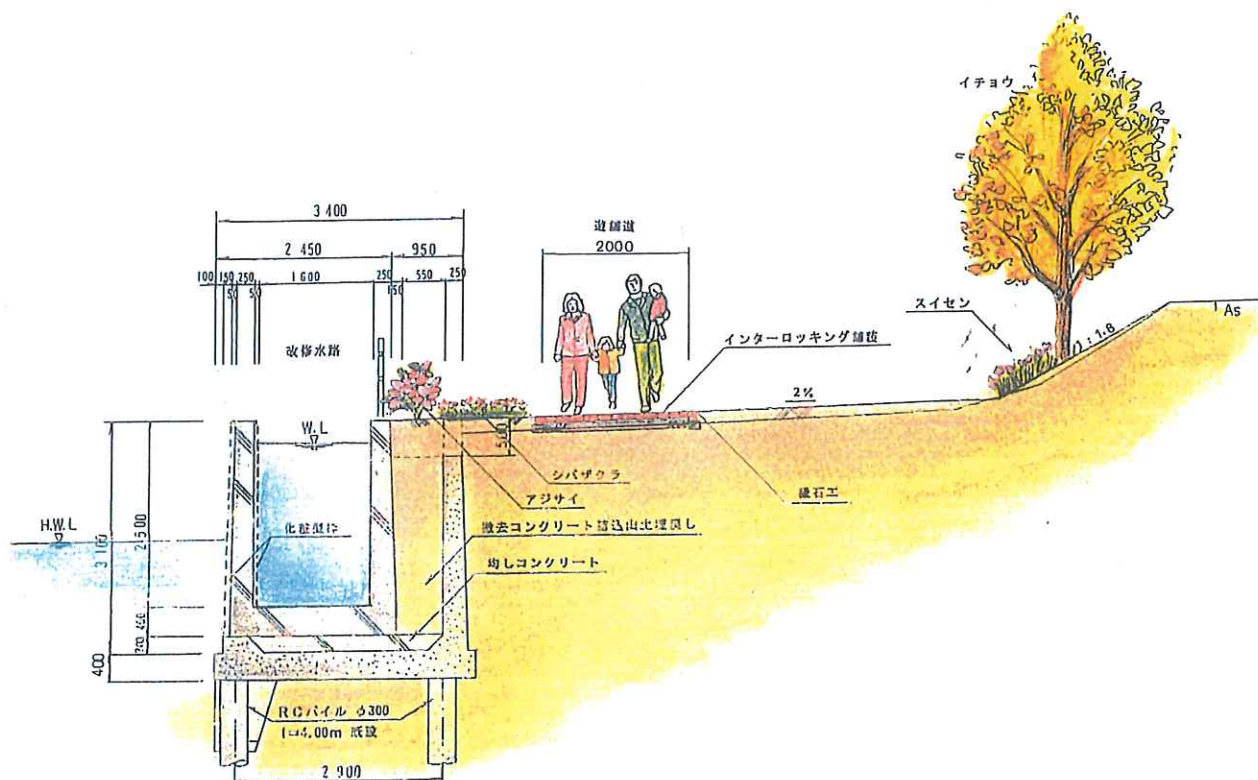
大阪府営いきいき水路「番田地区」断面イメージ図
