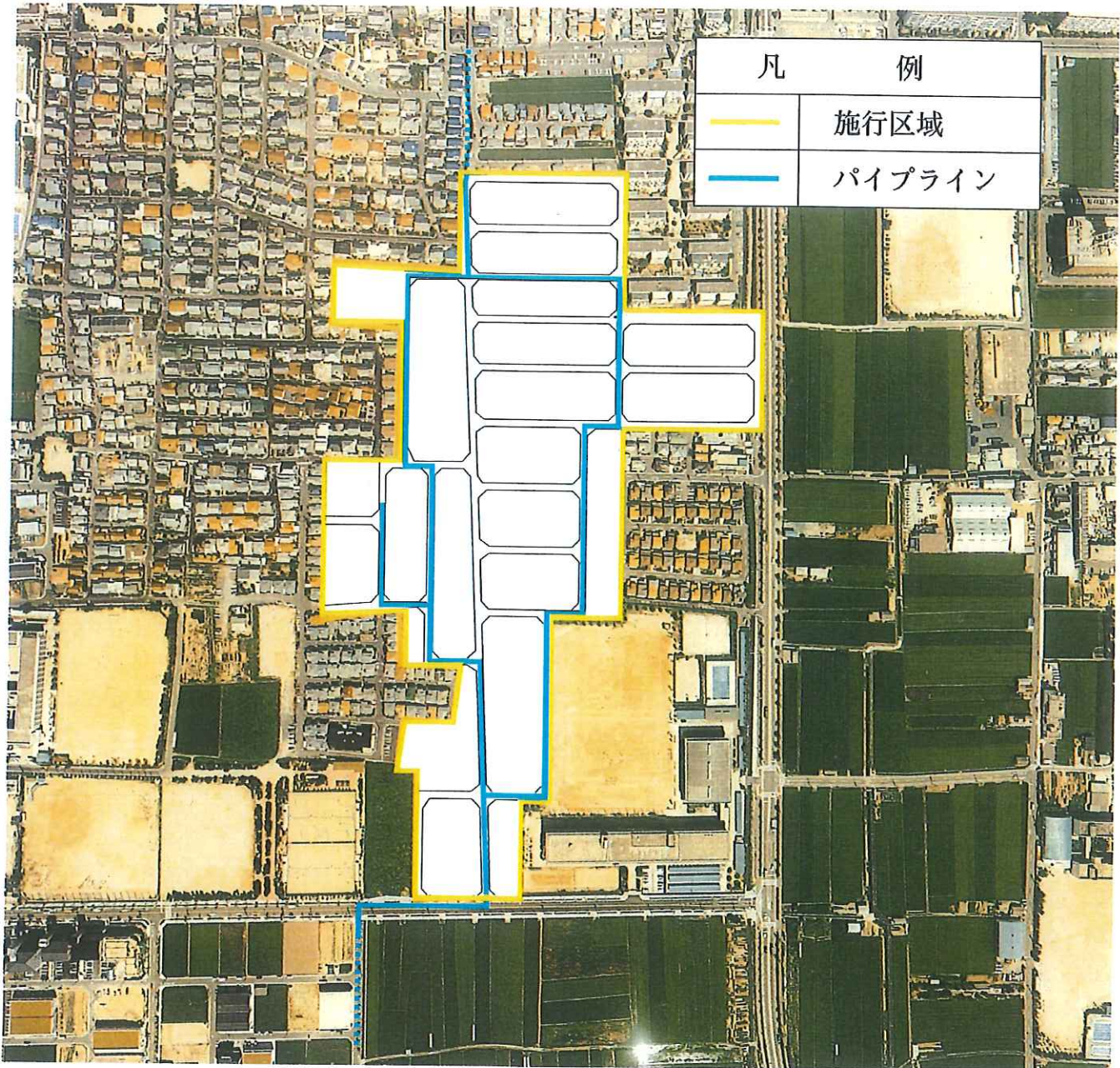
茨木市内瀬東土地区画整理事業区域内用水パイプライン
