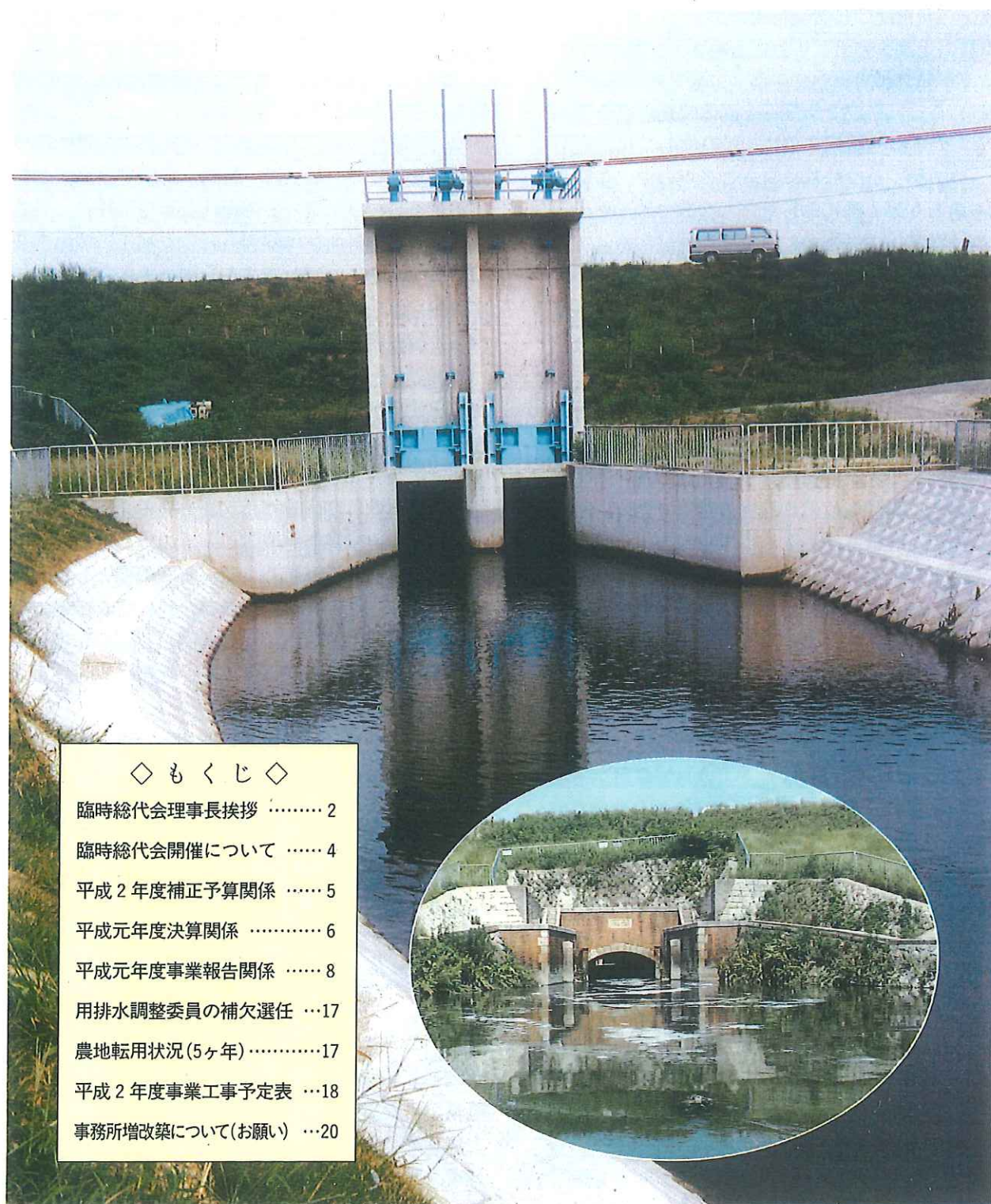
芥川引堤工事に伴い改築された芝生大樋
