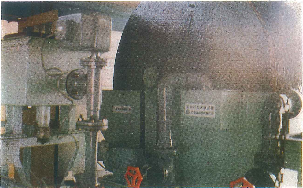
昭和52～53年度回転円盤（直径2.0m）実験装置
