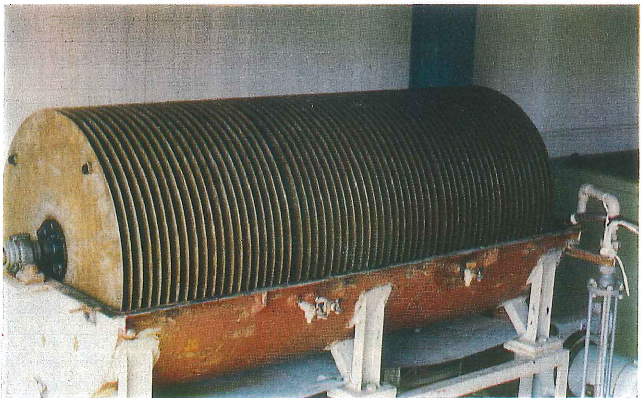
昭和51年度回転円盤（直径0.5m）実験装置
